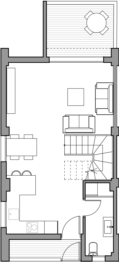
PLANTA BAJA
